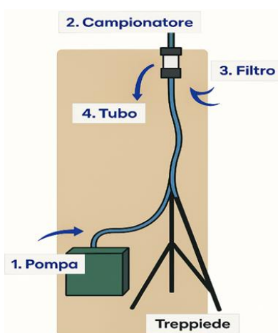
Figura 50 - campionatore ambientale o statico (schema)
